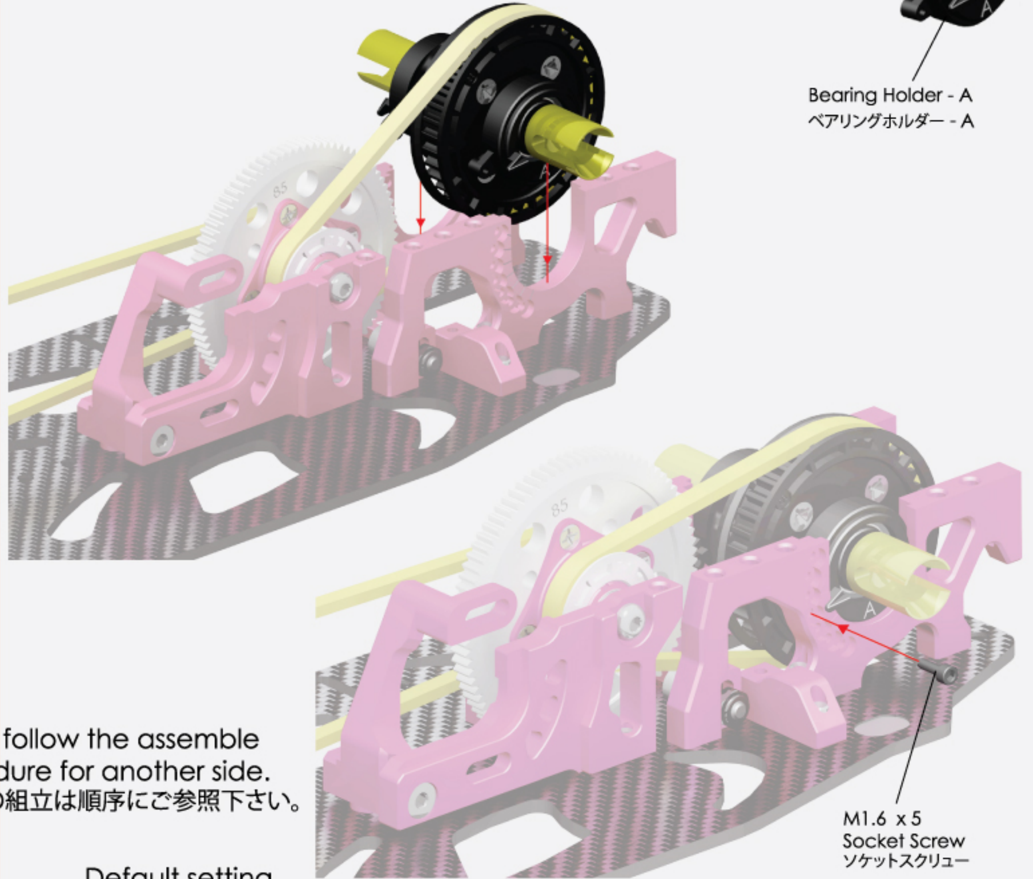
M1.6 x 5 Socket Screw (2) M1.6 x 5 ソケットスクリュー (2)
