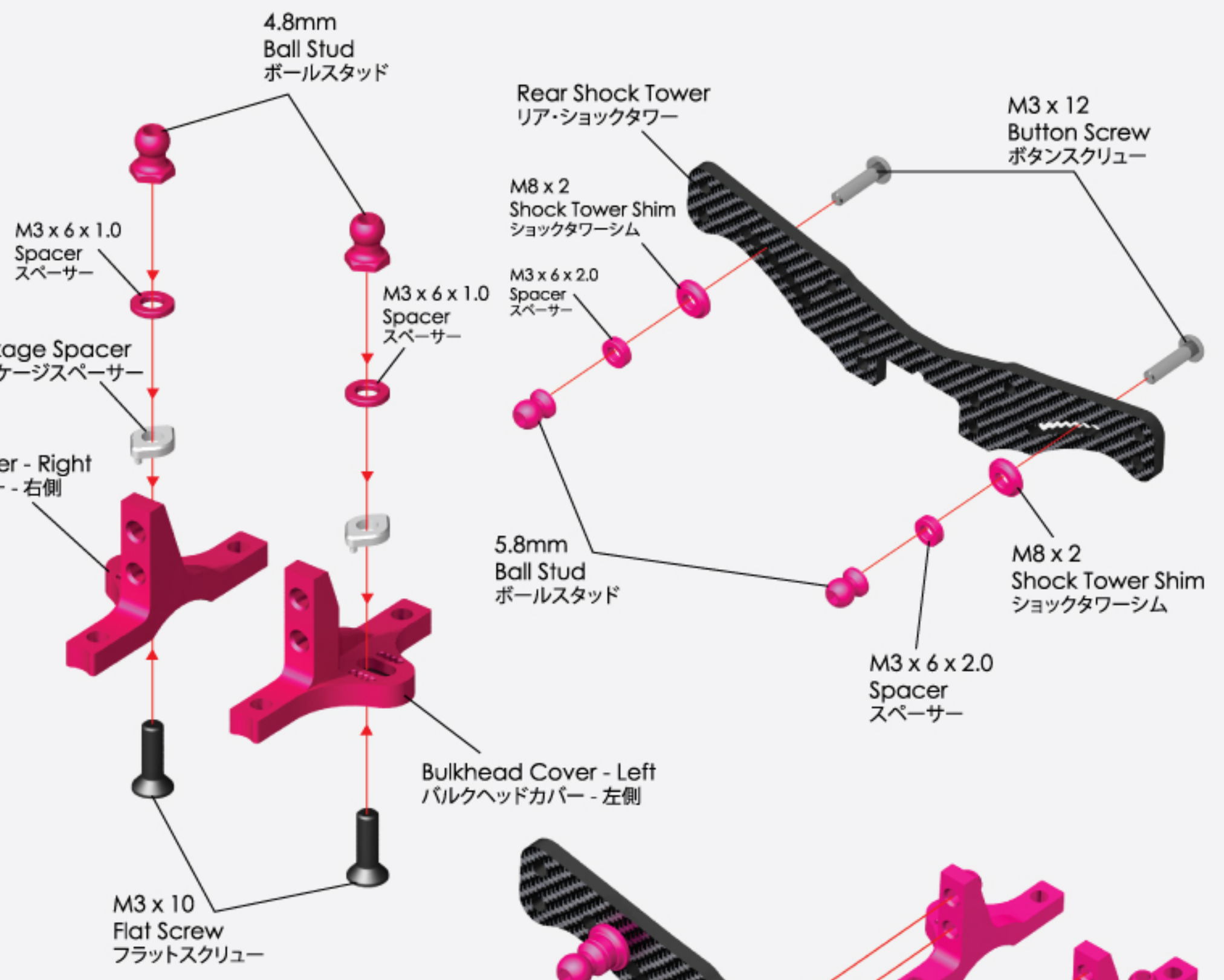
Upper Linkage Spacer (2) アッパーリンケージスペーサー (2)
