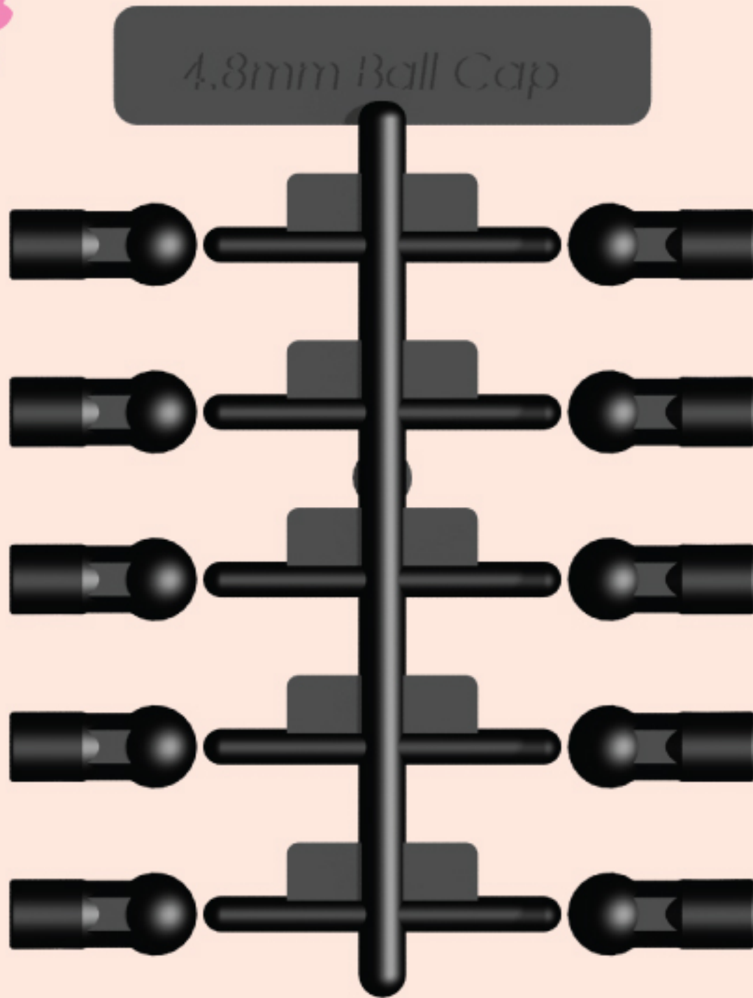
4.8mm x 12mm Ball Cap Set (1) 4.8mm x 12mm ボールキャップセット (1)
