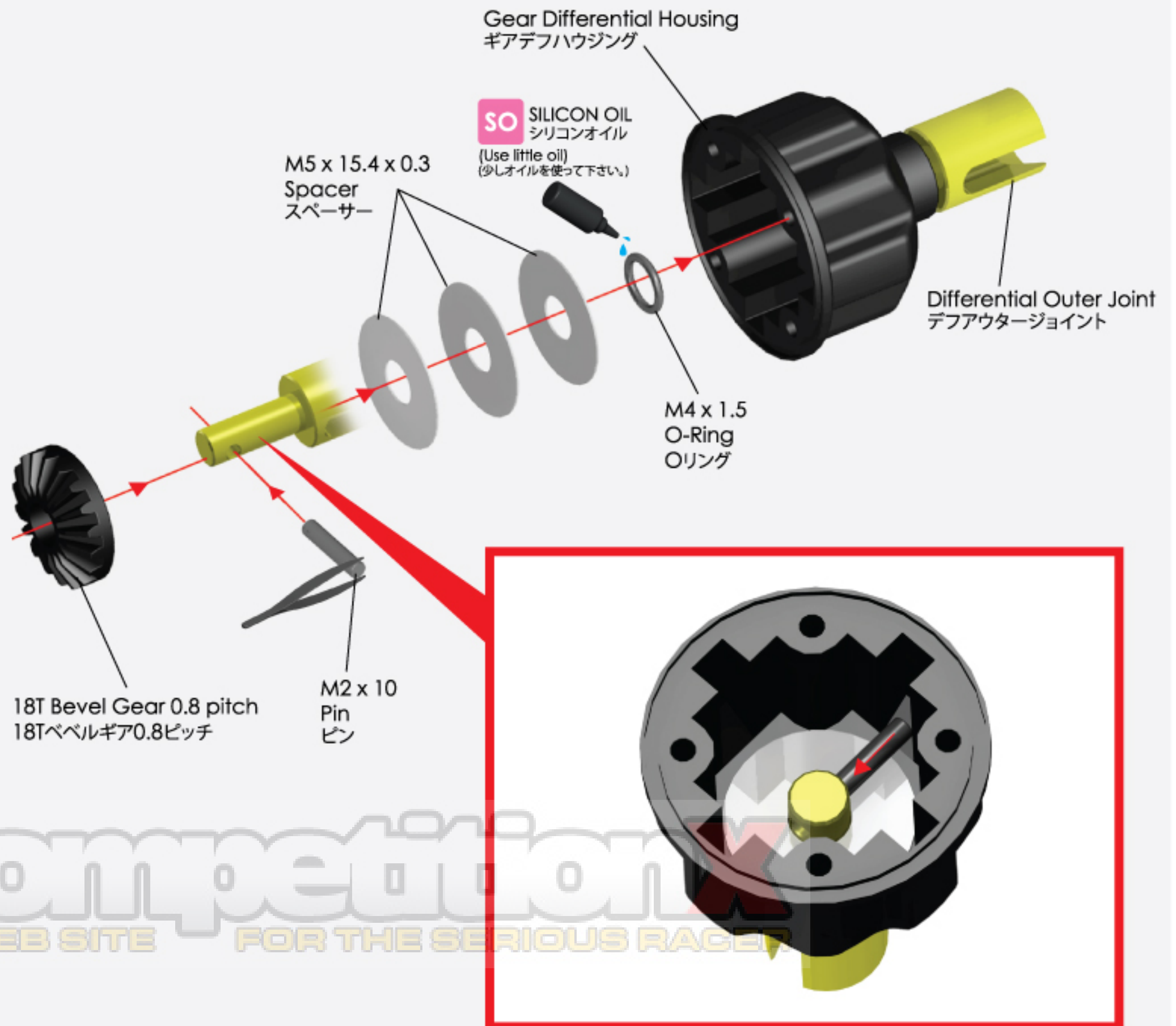
18T Bevel Gear 0.8 pitch (2) 18Tベベルギア0.8ピッチ (2)
