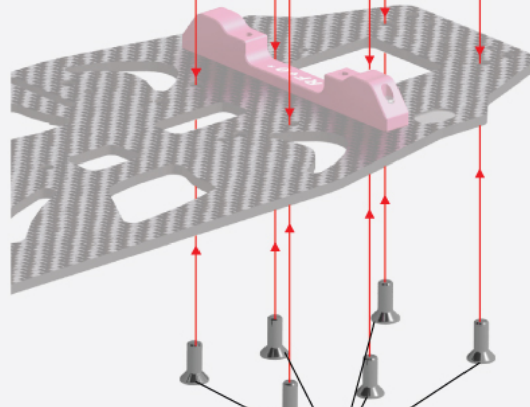
M3 x 8 Flat Screw フラットスクリュー
