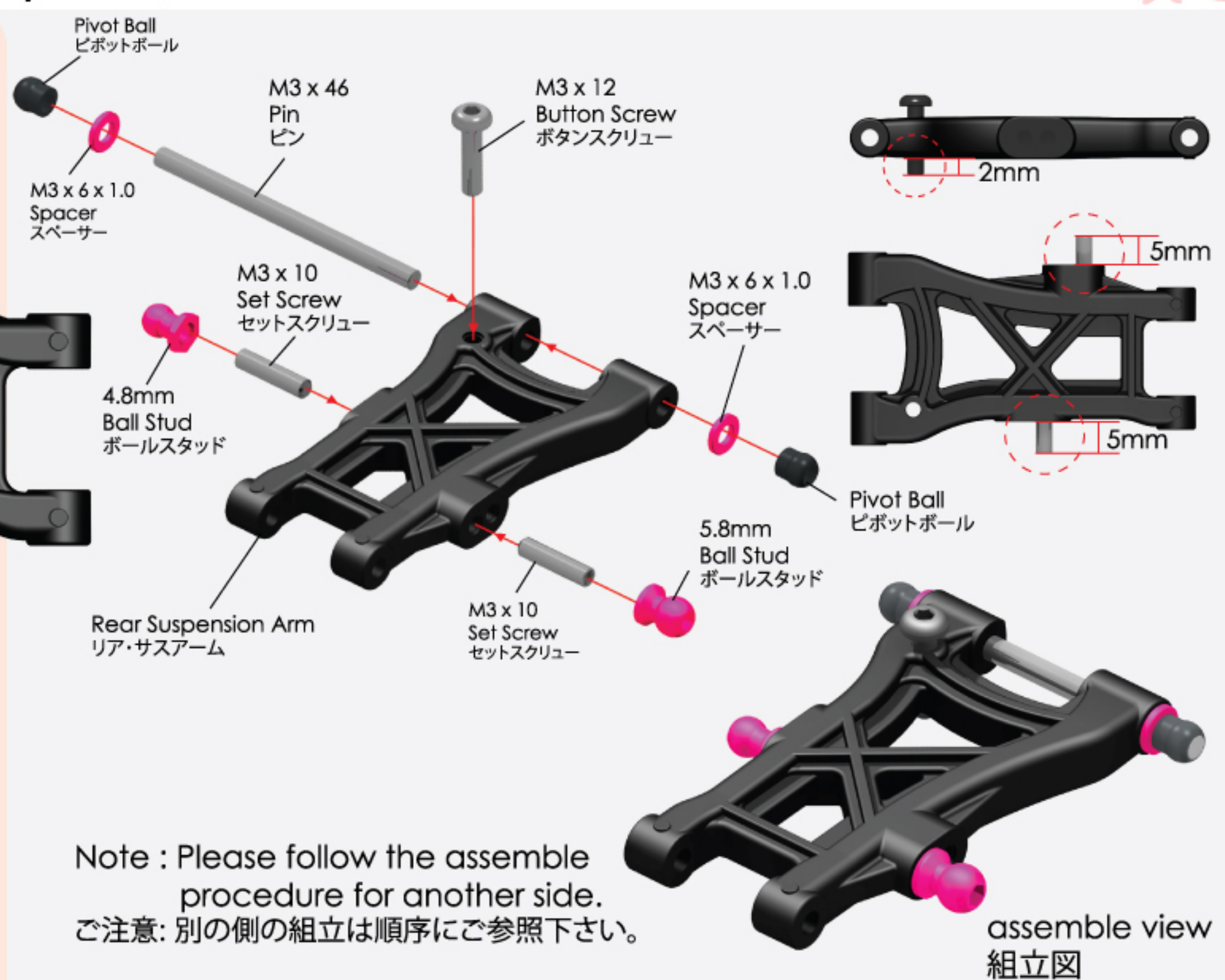
Rear Suspension Arm (2) リア・サスアーム (2)
