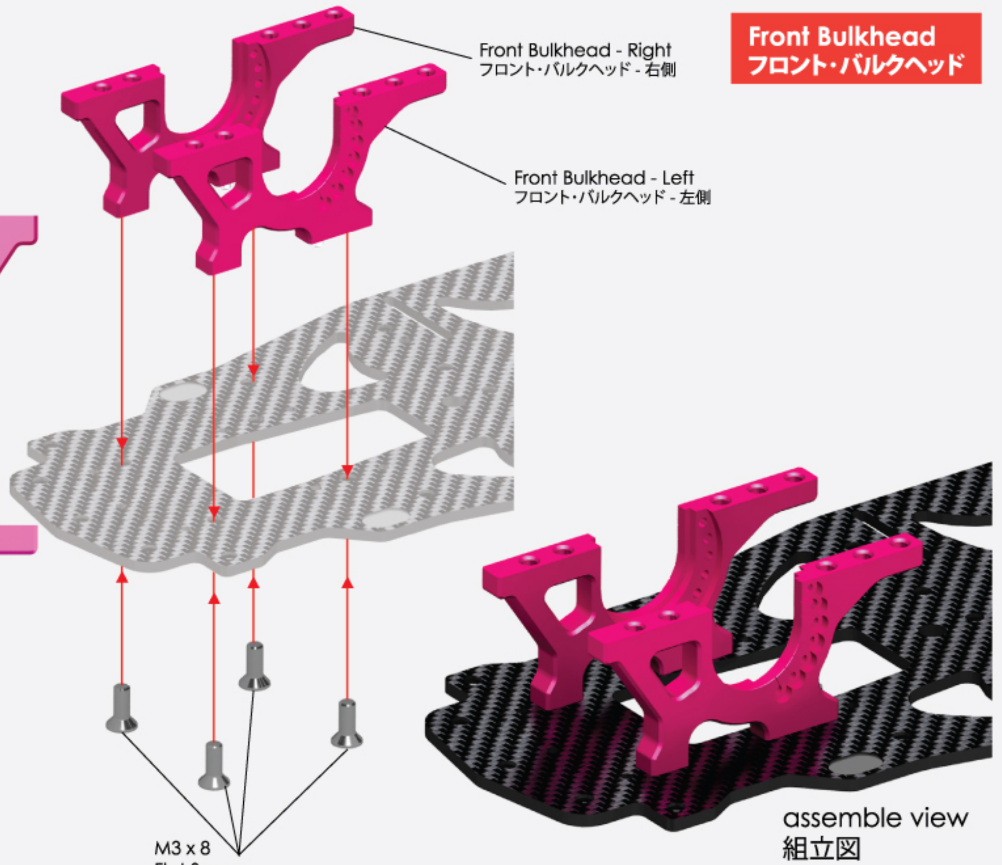
Front Bulkhead - Right (1) フロント・バルクヘッド - 右側 (1)
