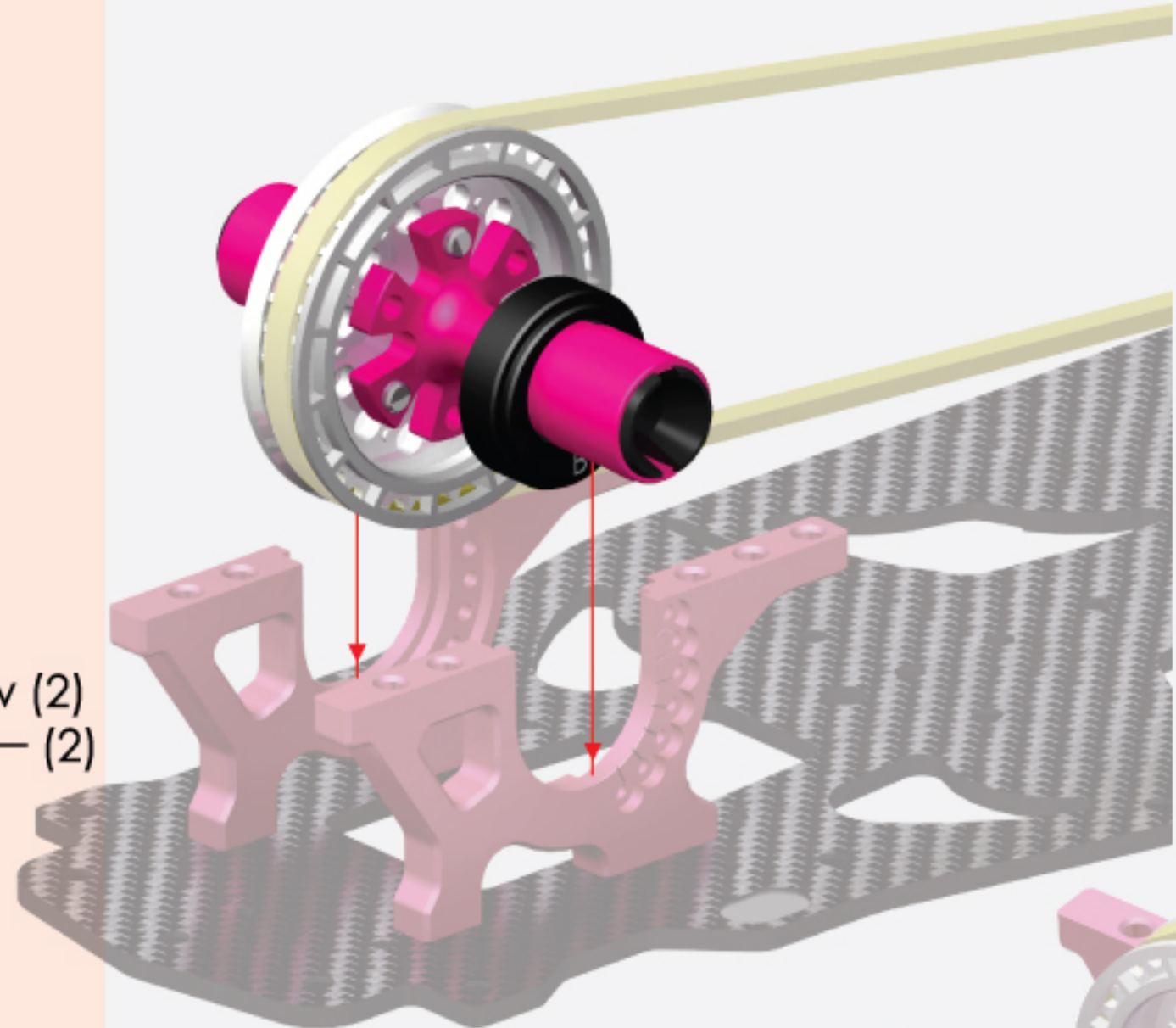
Bearing Holder - A(1) ベアリングホルダー - A(1)
