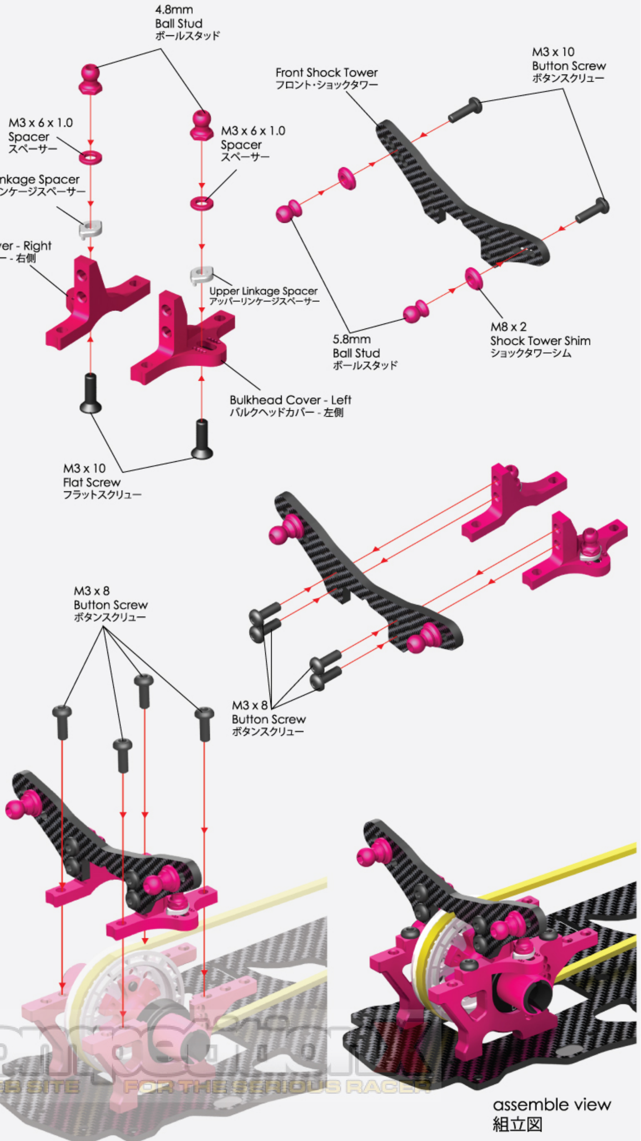
Upper Linkage Spacer (2) アッパー・リンケージスペーサー (2)
